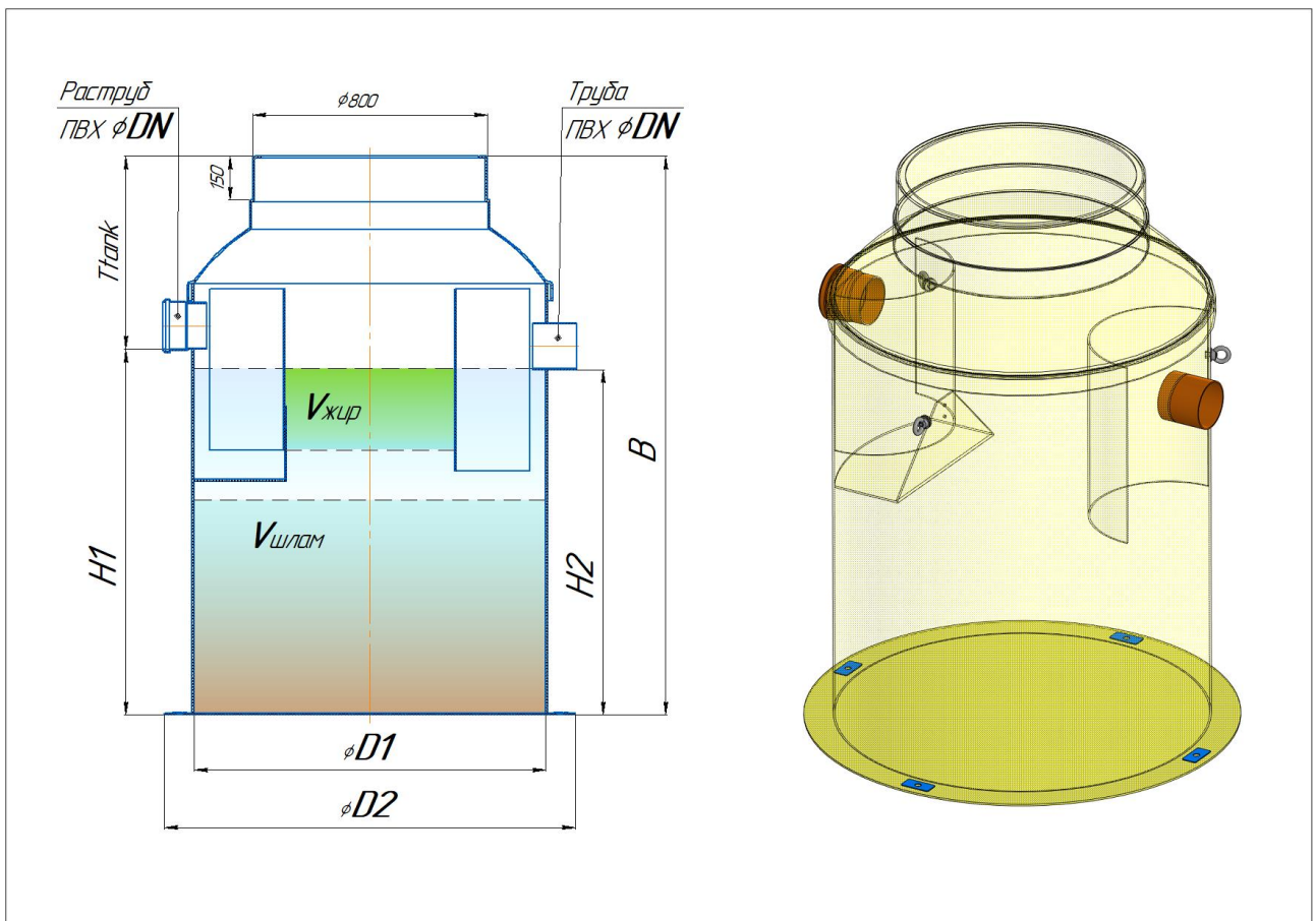
Рисунок 1 - Принципиальная схема установки Lipimax G-V
